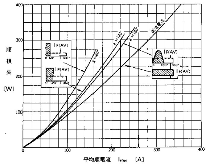
順損失
