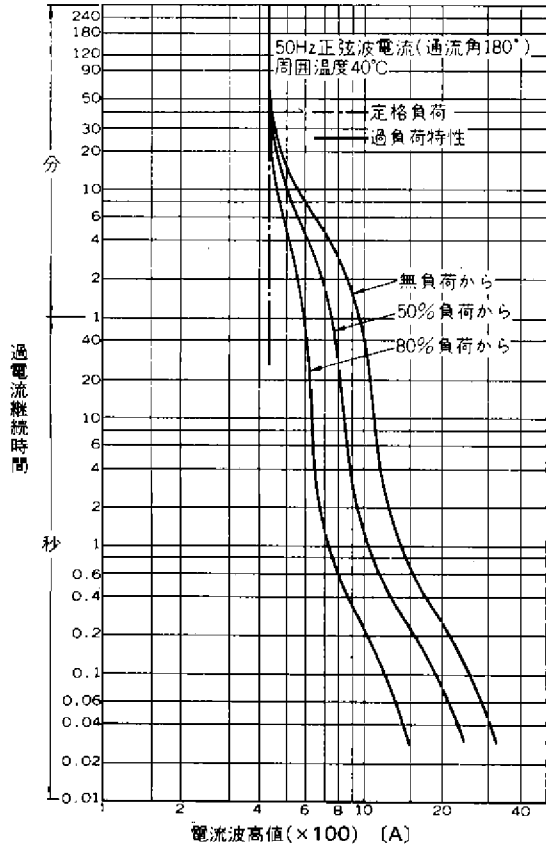
過負荷電流—時間 (冷却体AL01-20自冷)
