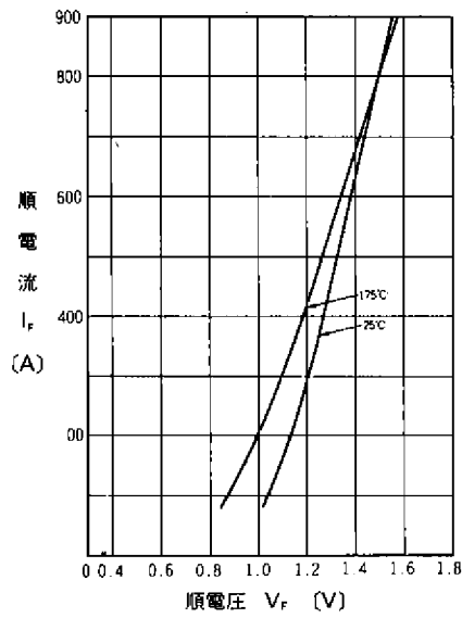
順特性
