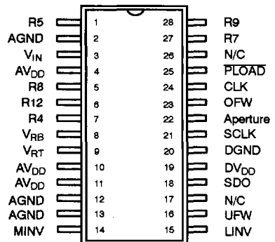
28 Pin SOIC (Jedec, 0.300")
