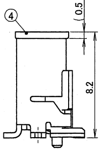
キャップ装着状態 /With CAP
