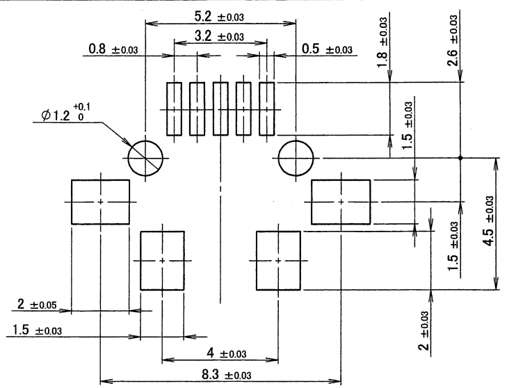
推奨基板寸法 RECOMMEND PCB LAYOUT
