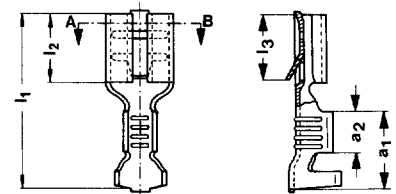
Schnitt A - B
