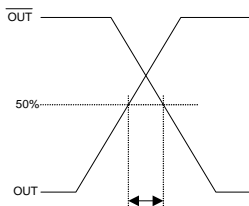
LVPECL Output Skew
