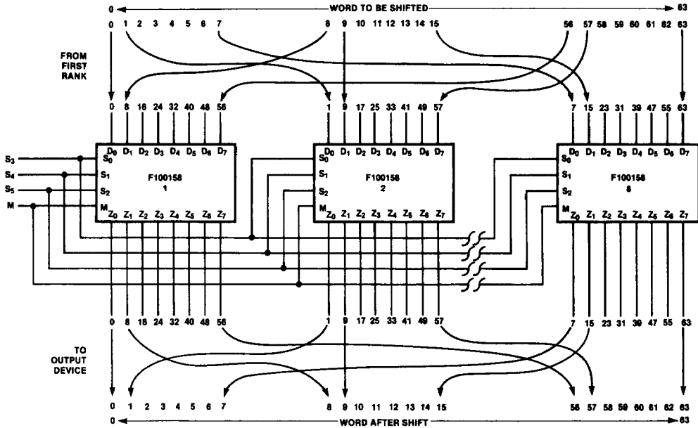
FIGURE 5. Modulo-8 Shift
