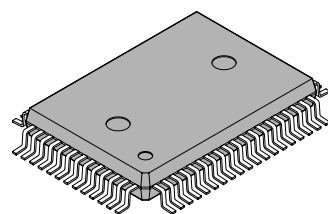
(FPT-64P-M06)
