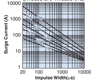
Image Derating (NVD20U-270~NVD20U-910)
