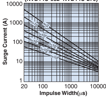
Image Derating (NVD14U-082~NVD14U-270)
