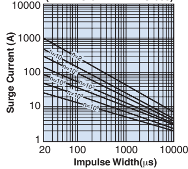
Image Derating (NVD14U-082~NVD14U-270)
