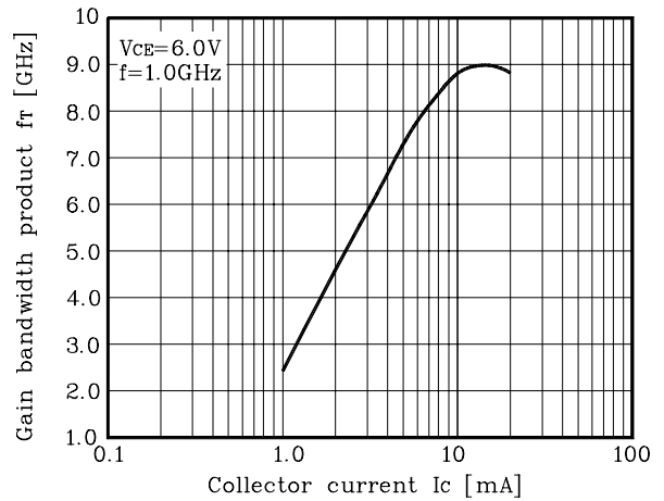
Fig. 4 f_T-I_C
