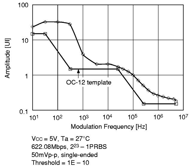
Fig. 13. Jitter tolerance
