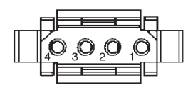
Receptacle
