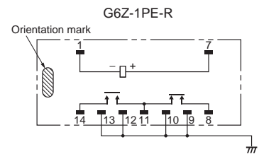
G6Z-1PE-R
