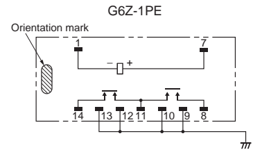
G6Z-1PE
