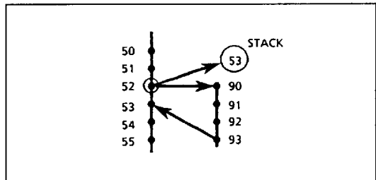
Figure 4: COND JSB PL (CJS)
