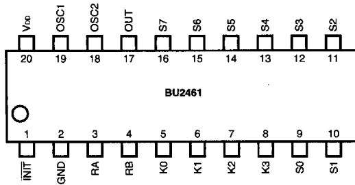
BU2461 pin layout
