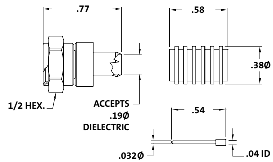
DataGrade RG-6/U FD
