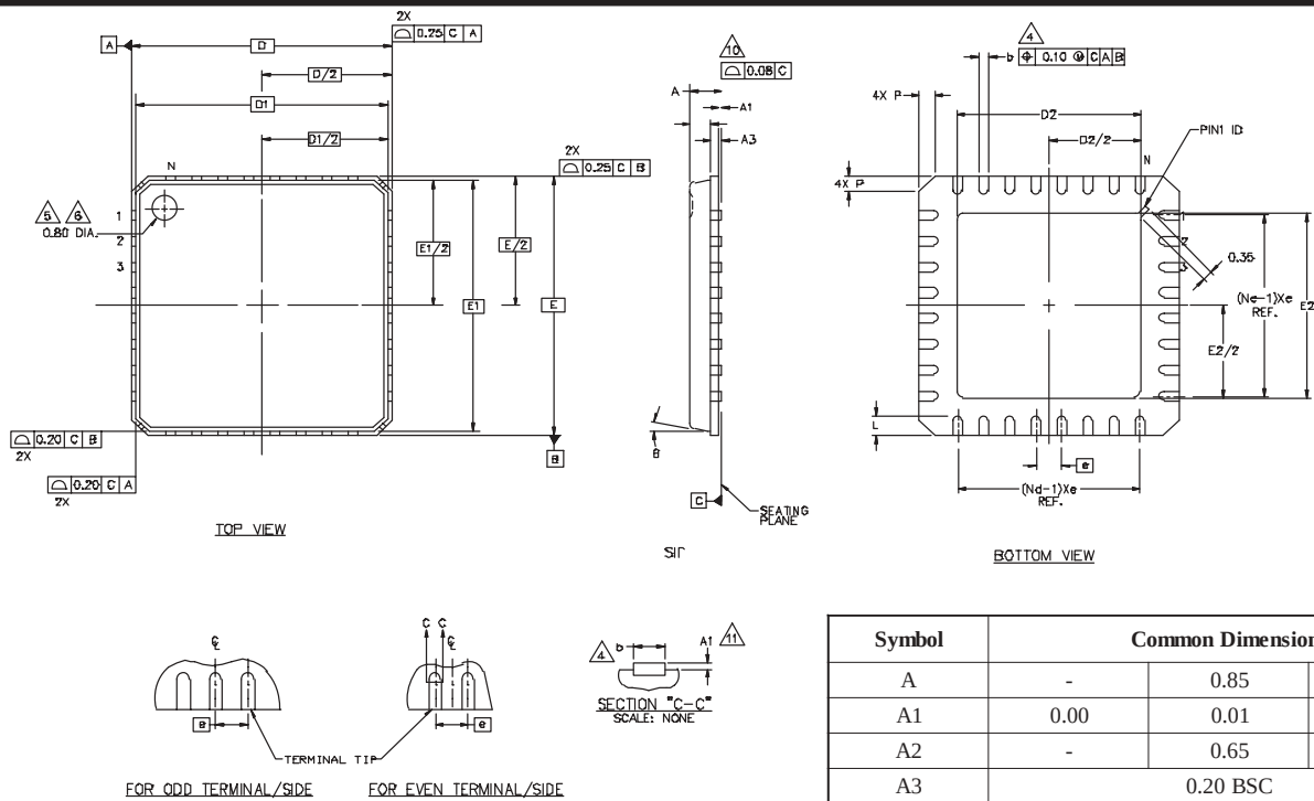
56 pin MLF2
