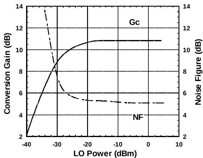
Gc, NF vs. LO Power
