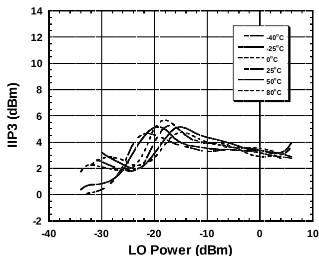
IIP3 vs. LO Power
