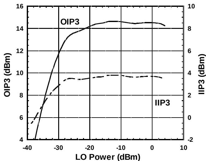
OIP3, IIP3 vs. LO Power
