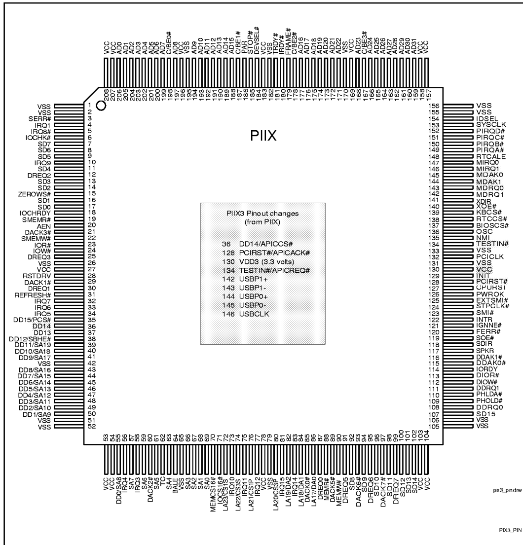
Figure 11. PII/PIIX Pin Assignment
