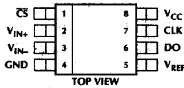
ML2281 8-Pin SOIC
