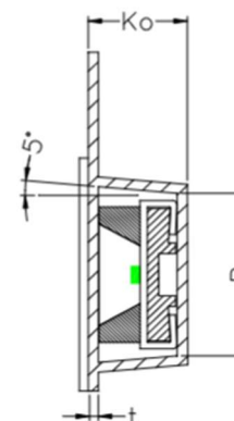
SEC:A-A'
