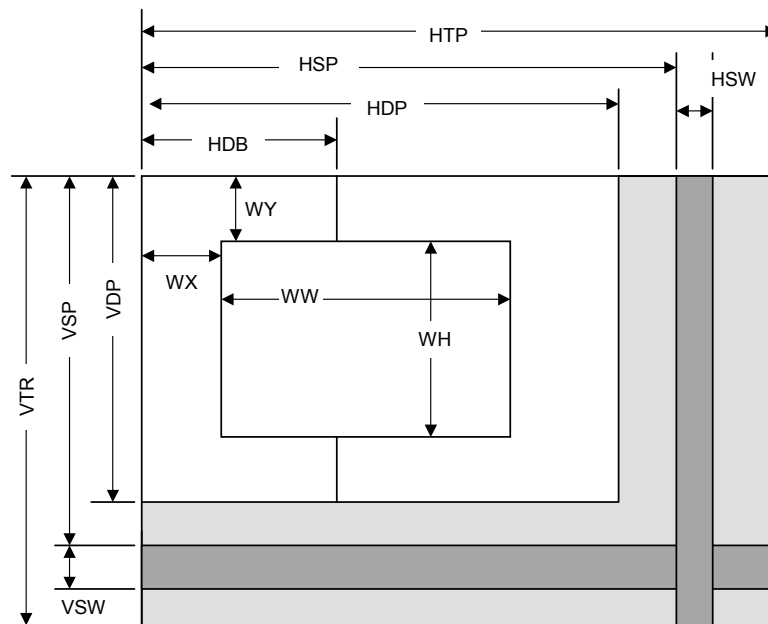
Fig. 5.1 Display Parameters
