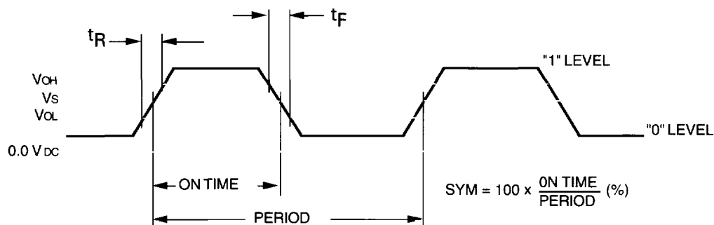
Figure 2. Waveform Parameters
