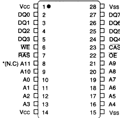
28Pin Plastic SOJ (300mil)
