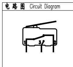
示意图 CHEMATIC
