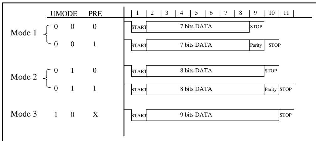
Fig. 5-12 UART Mode
