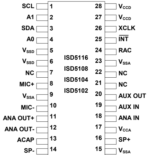
SOIC
