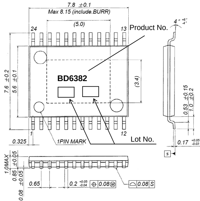
HTSSOP-B24 (Unit:mm)
