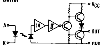
OPB10510/OPB10530 (Totem-Pole Output) Buffer
