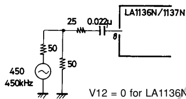
IF input
