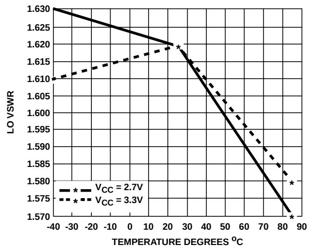
FIGURE 45. LO 50Ω VSWR
