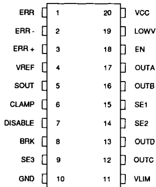
20-Pin DIP, SO
