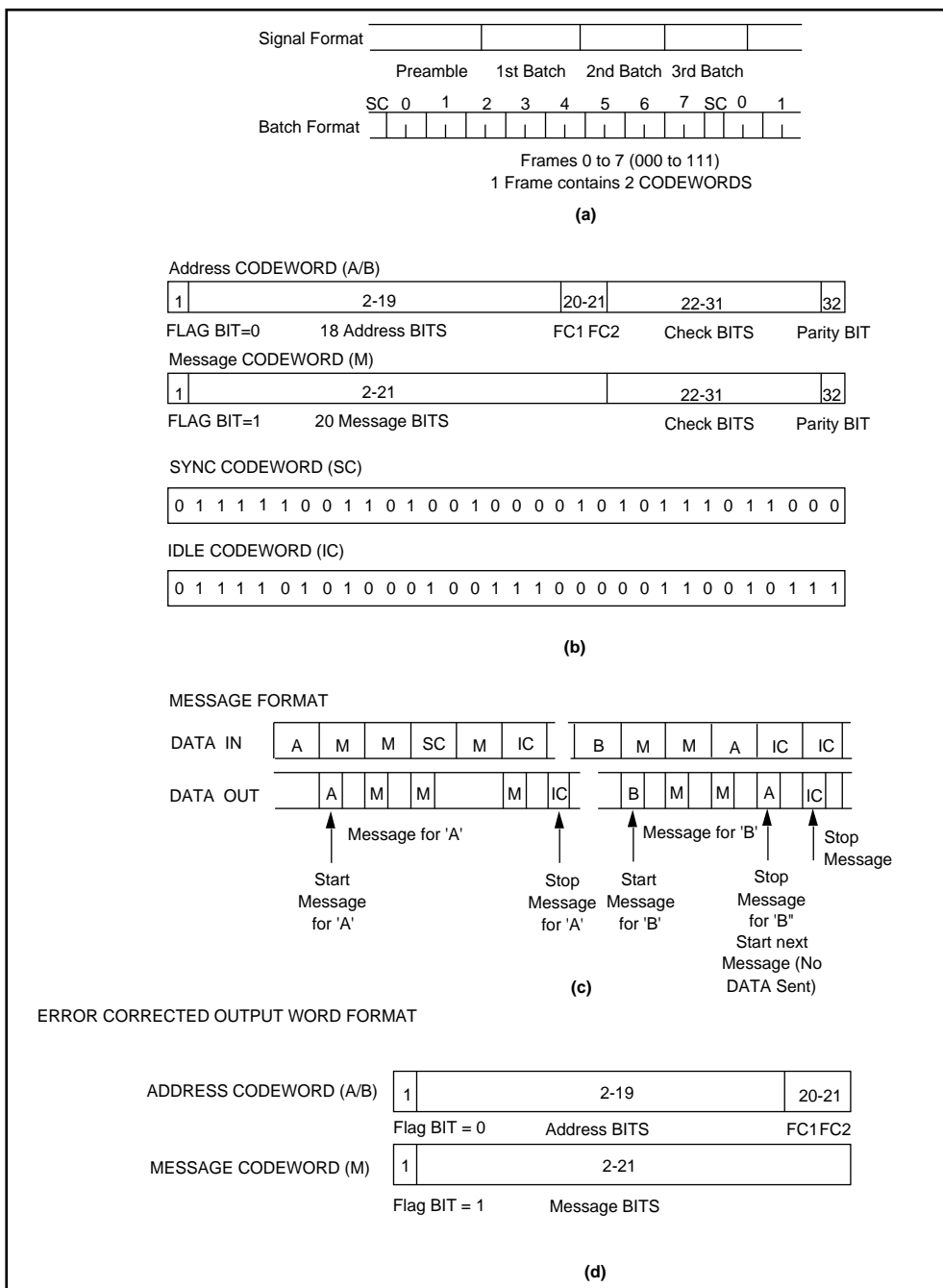
Fig. 3 POCSAG Data Format
