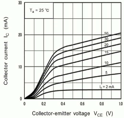
Fig. 11.8 I_C - V_{CEO}
