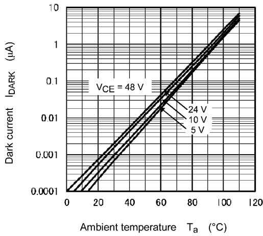
Fig. 11.9 I_{\text{DARK}} - T_a
