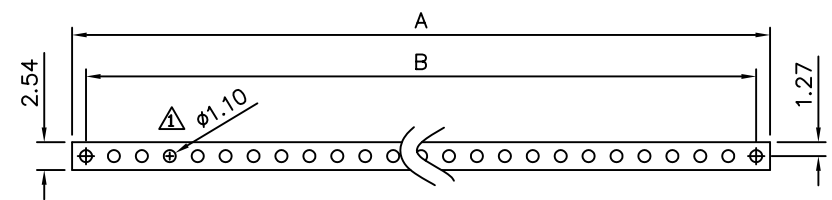
P.C.B Layout
