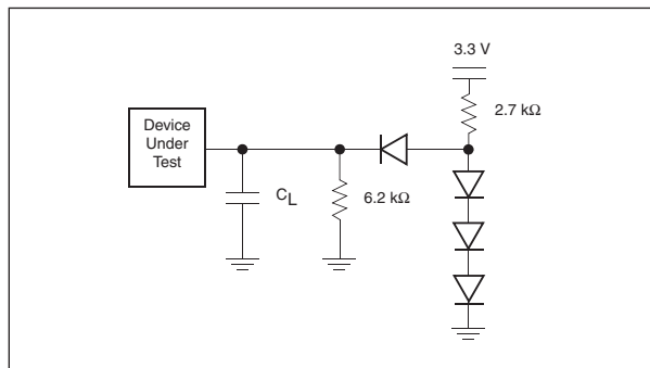
FIG: 4 TEST SETUP
