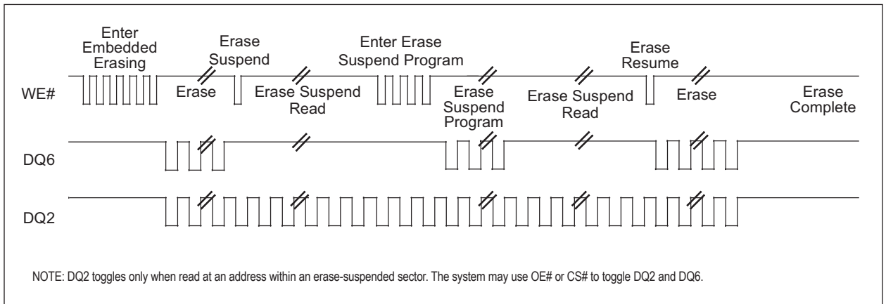
FIG 25: DQ2 VS. DQ6
