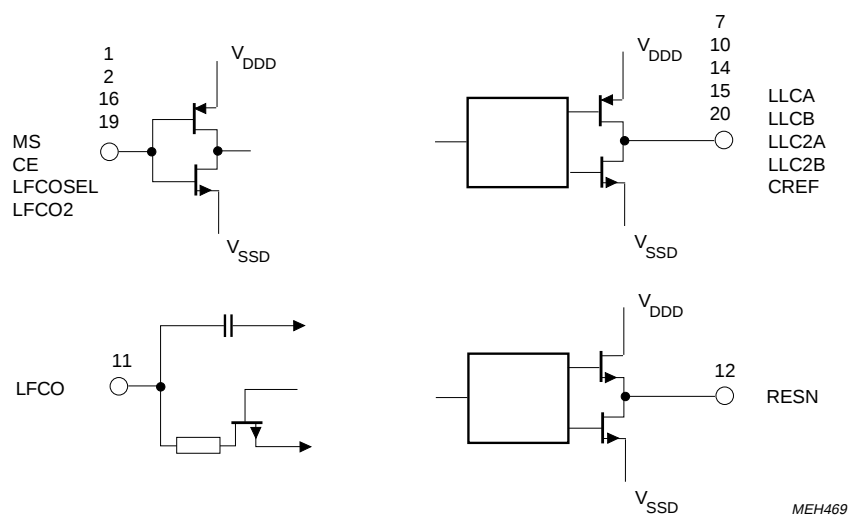
Fig.5 Internal circuit.
