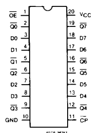
CD54/74AC/ACT534
