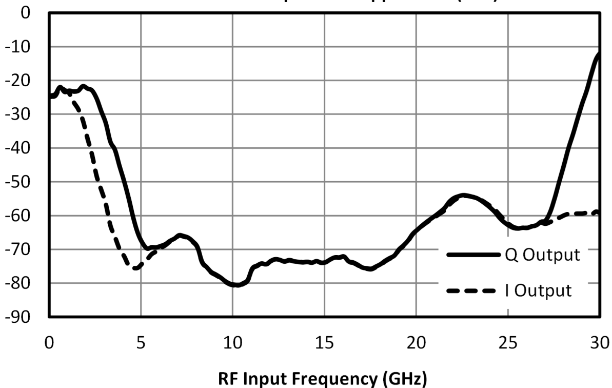
2RF x 0LO Spurious Suppression (dBc)
