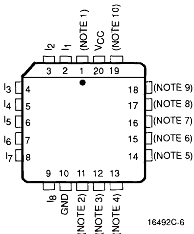
20-Pin PLCC
