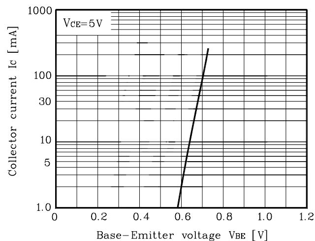
Fig. 2 I_C - V_{BE}
