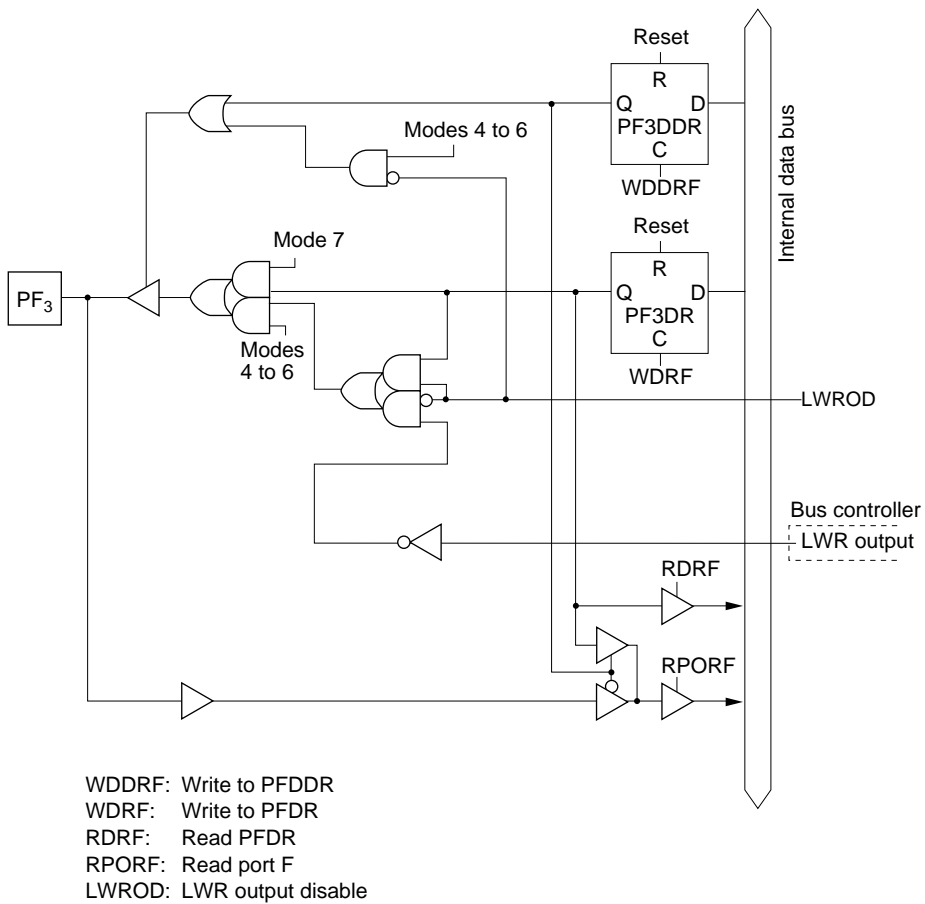
Figure 5.41 (d) Port F Block Diagram (Pin PF 3 )
