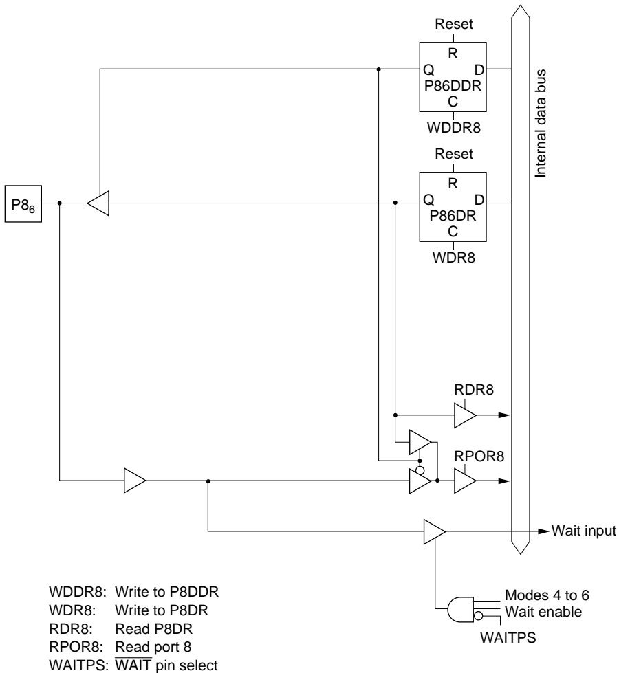
Figure 5.34 (d) Port 8 Block Diagram (Pin P8 6 )
