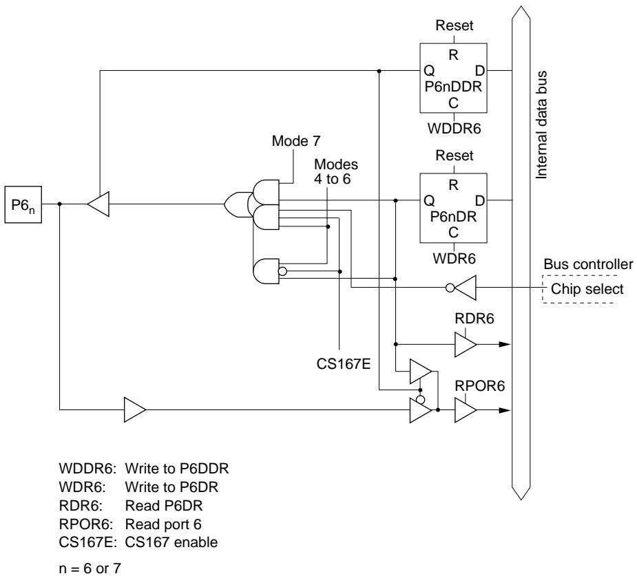
Figure 5.32 (d) Port 6 Block Diagram (Pins P6 6 and P6 7 )
