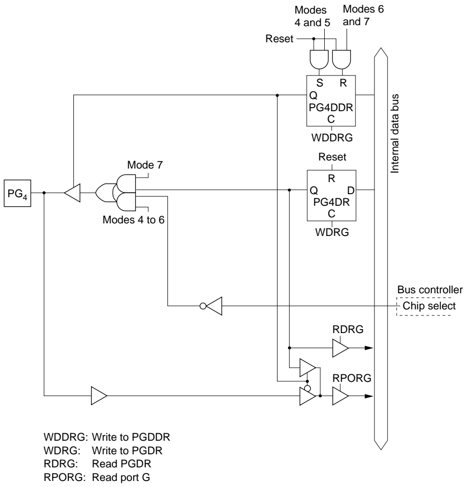
Figure 5.42 (d) Port G Block Diagram (Pin PG 4 )
