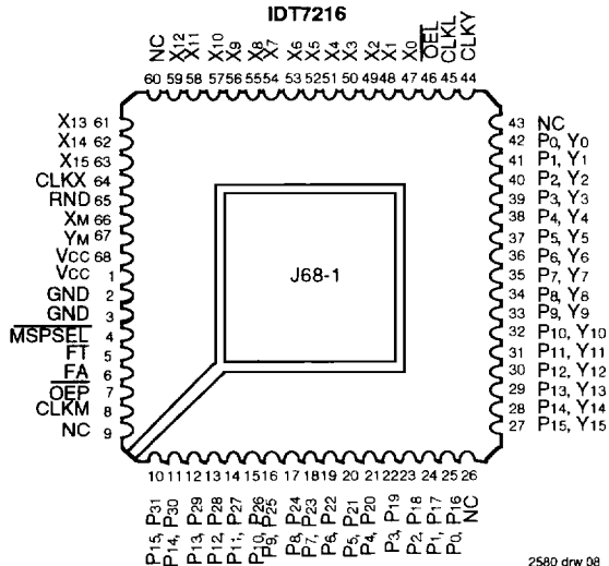
IDT7216
