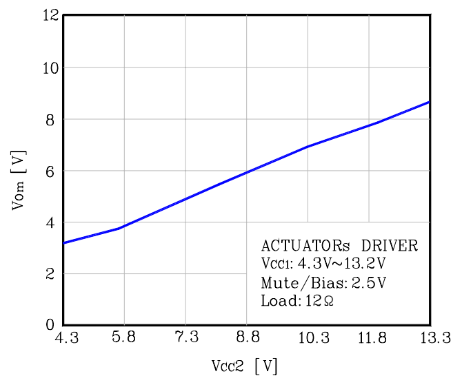
Fig. 4 V_{OM} - V_{CC}
