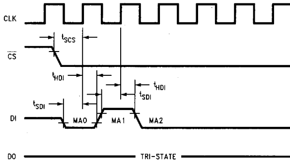
FIGURE 2. DI Timing
