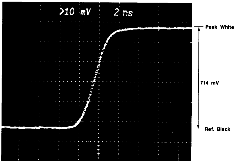
G Output Rising Edge
