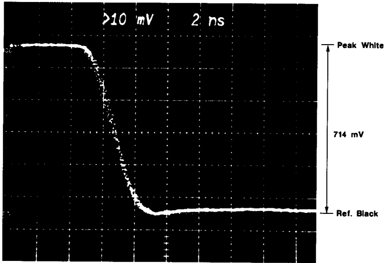
G Output Falling Edge
