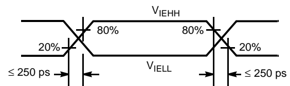
(d) LVPECL Input Test Waveform
