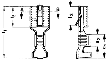
Schnitt A-B
