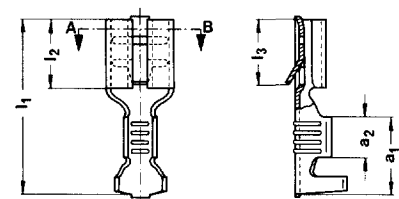
Schnitt A-B
