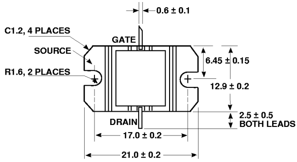
C21A Package Outline IM5053-4L and IM5053-8L
