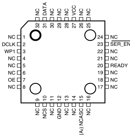
32 TQFP
