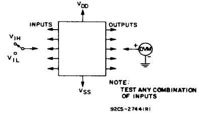
Fig. 16 - Input voltage.
